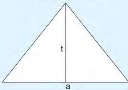
Segitiga sama sisi
