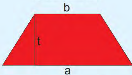
Trapesium sama kaki
