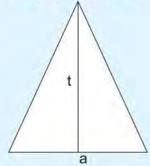
Segitiga sama kaki
